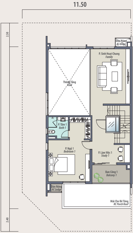
Mặt Bằng Tầng 2 Second Floor Plan
