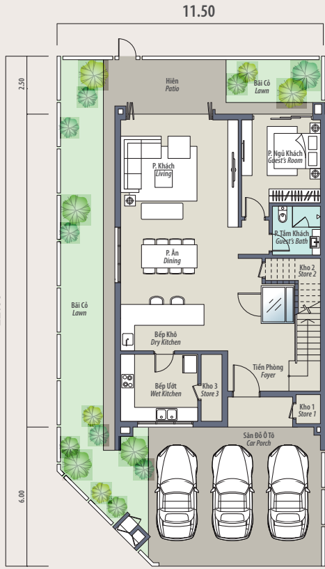
Mặt Bằng Tầng 1 First Floor Plan
