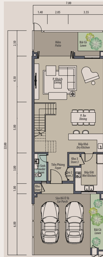
Mặt Bằng Tầng 1
