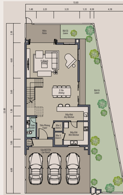
Mặt Bằng Tầng 1
