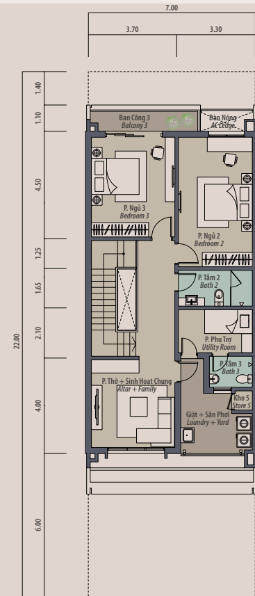
Mặt Bằng Tầng 3
