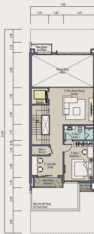
Mặt Bằng Tầng 2
