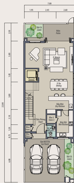
Mặt Bằng Tầng 1
