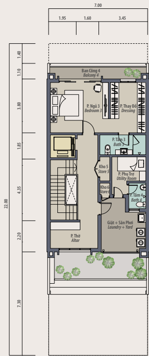
Mặt Bằng Tầng 4
