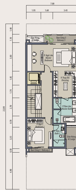
Mặt Bằng Tầng 3
