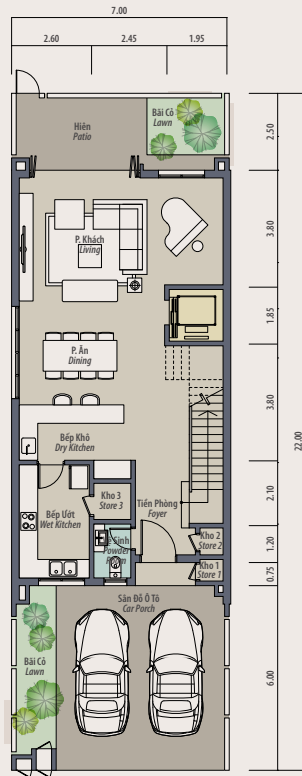
Mặt Bằng Tầng 1
