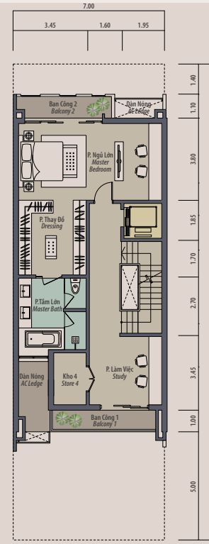
Mặt Bằng Tầng 3
