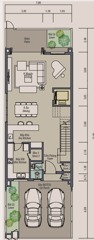
Mặt Bằng Tầng 1
