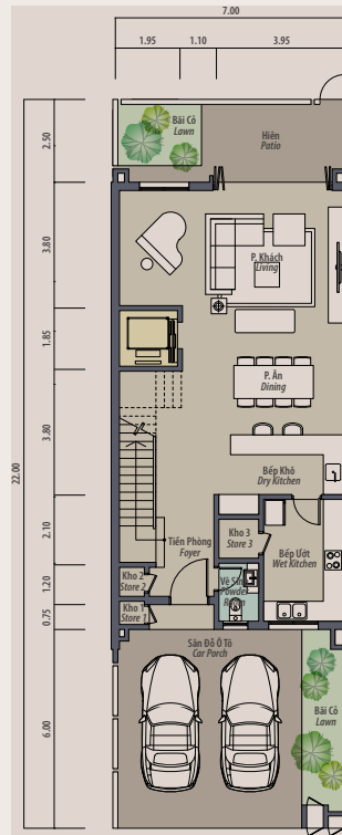
Mặt Bằng Tầng 1
