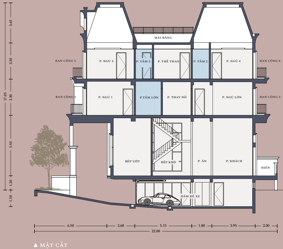
▲ MẶT CẮT
