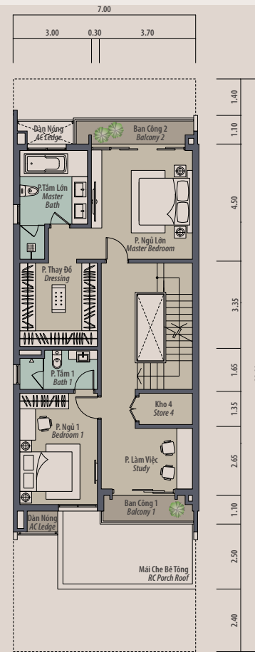
Mặt Bằng Tầng 2 Second Floor Plan
