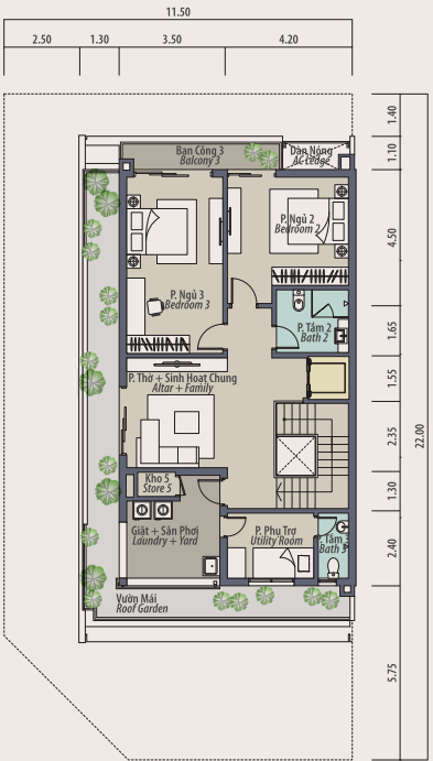
Mặt Bằng Tầng 3 Third Floor Plan
