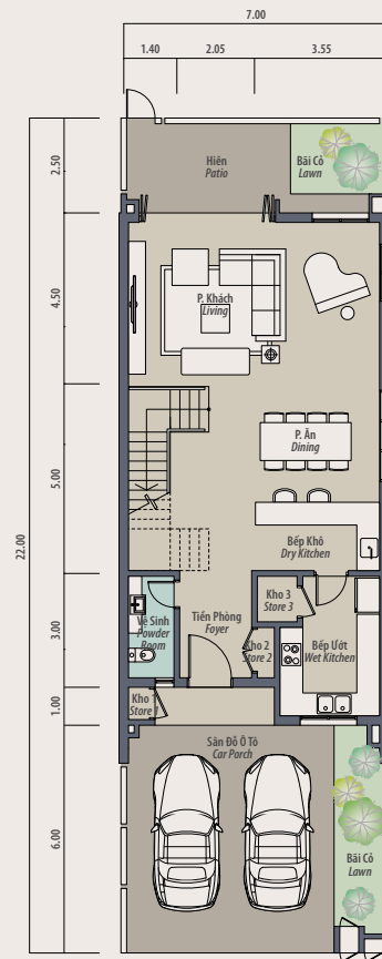
Mặt Bằng Tầng 1 First Floor Plan
