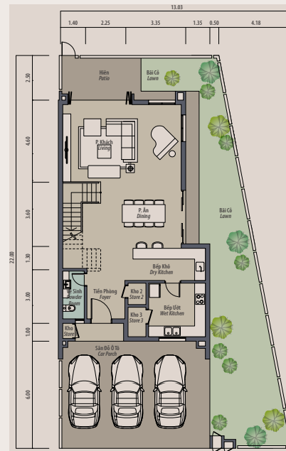
Mặt Bằng Tầng 1 First Floor Plan
