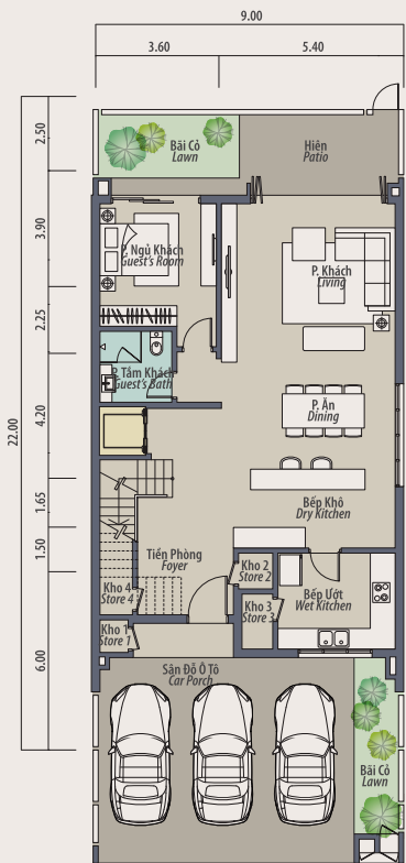
Mặt Bằng Tầng 1 First Floor Plan
