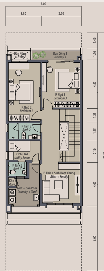
Mặt Bằng Tầng 3 Third Floor Plan
