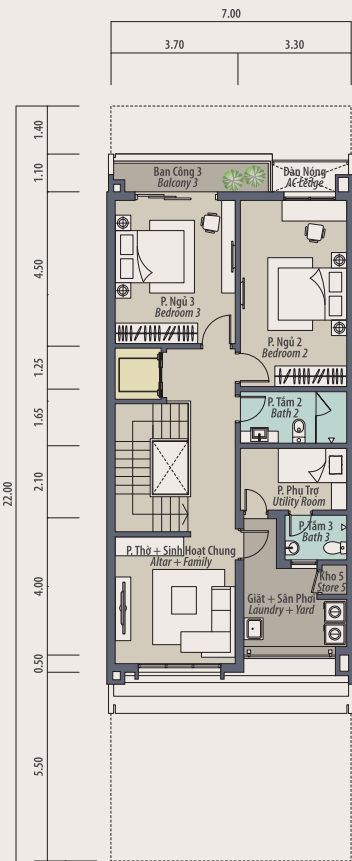
Mặt Bằng Tầng 3 Third Floor Plan
