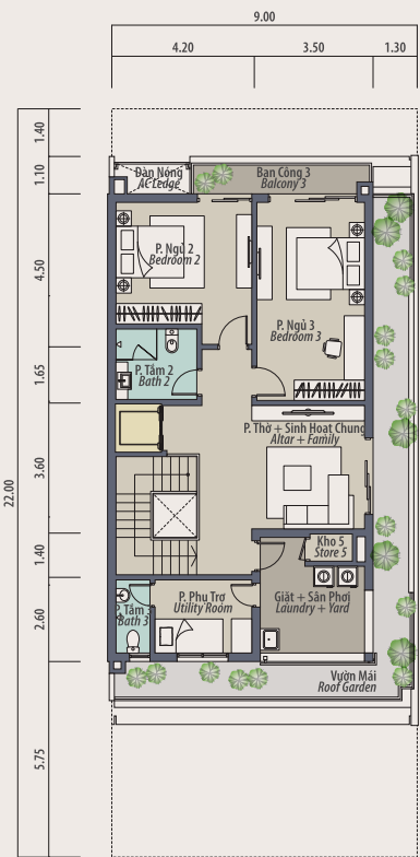
Mặt Bằng Tầng 3 Third Floor Plan
