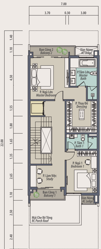
Mặt Bằng Tầng 2 Second Floor Plan
