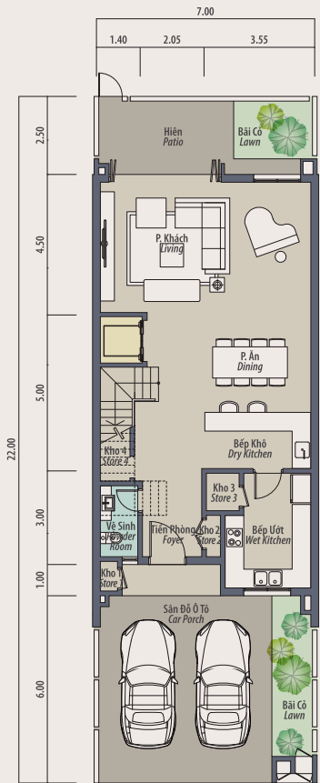
Mặt Bằng Tầng 1 First Floor Plan
