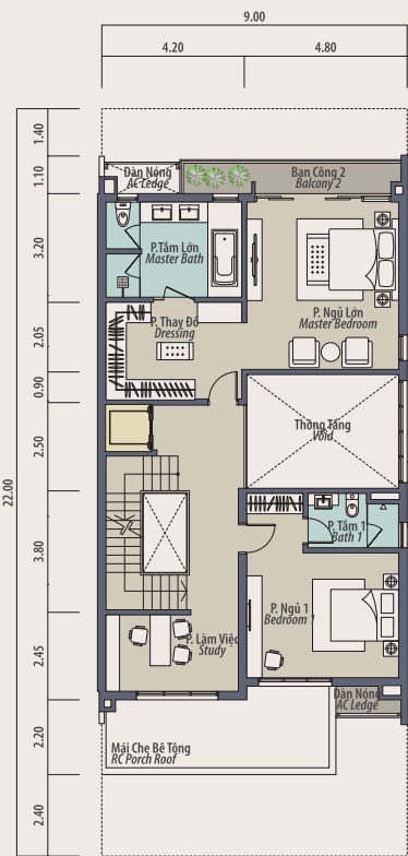
Mặt Bằng Tầng 2 Second Floor Plan
