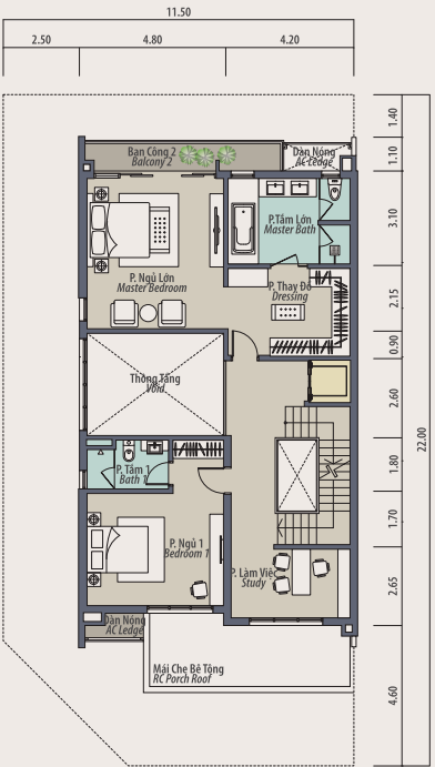
Mặt Bằng Tầng 2 Second Floor Plan
